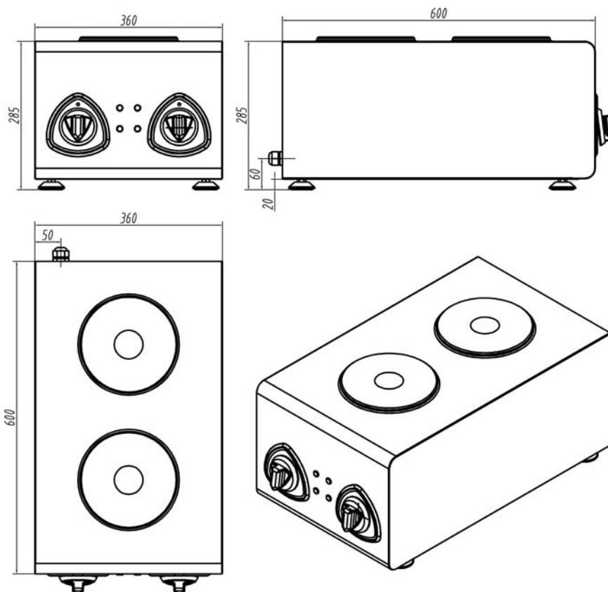
Модель 4B13.
